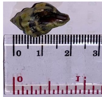
Species : Morula granulata
