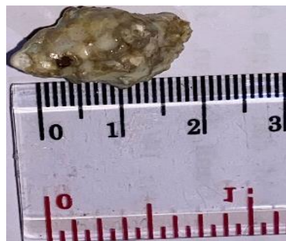
Spesies : Hexaplex trunculus
