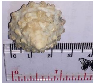
Spesies : Mitrella scripta
